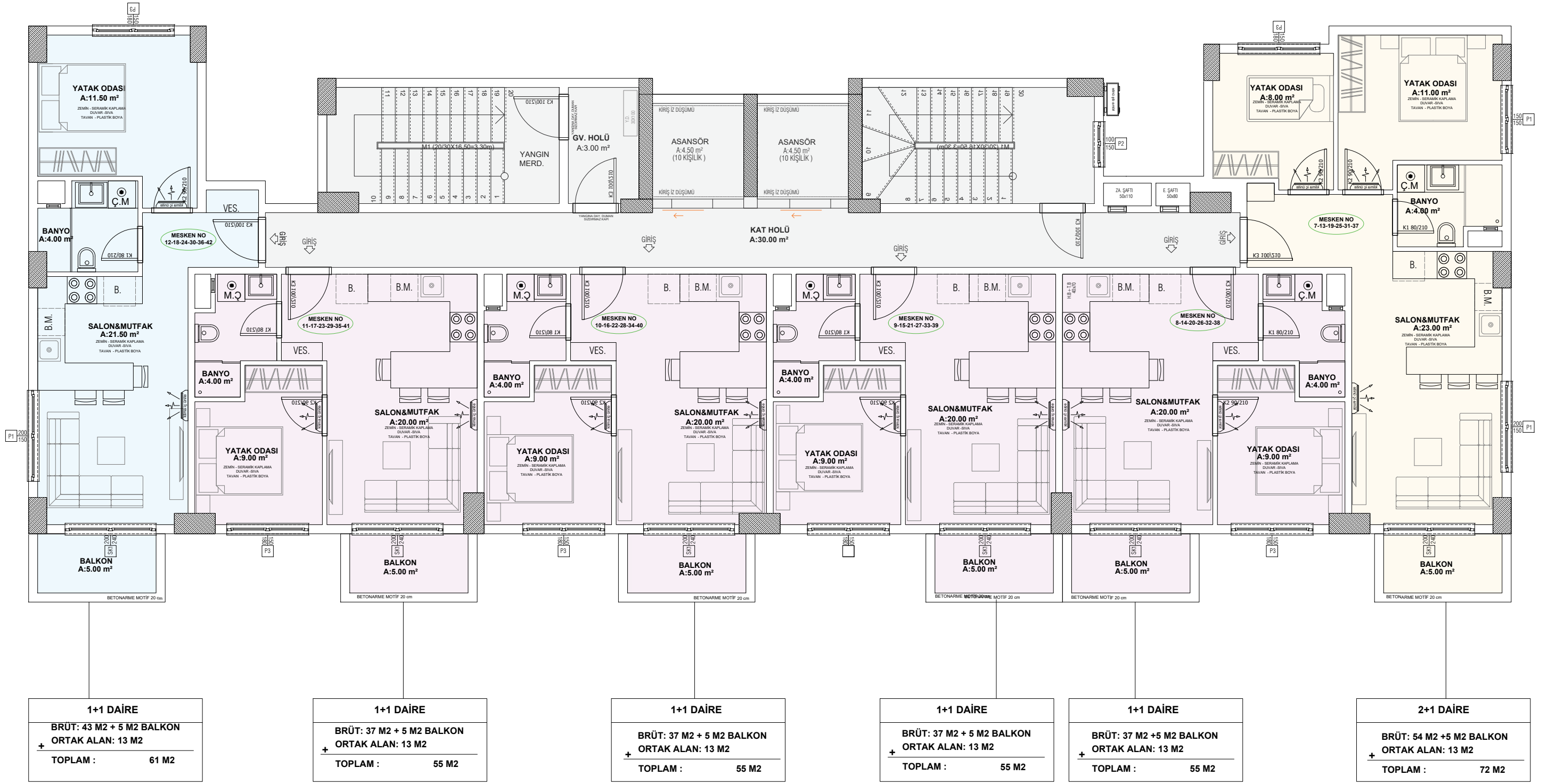
A BLOK TİP KAT PLANI
